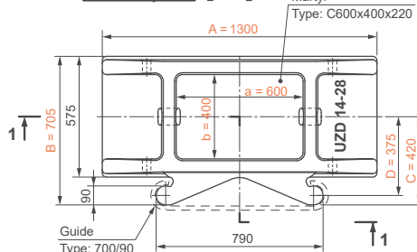
Vue en plan [mm]
