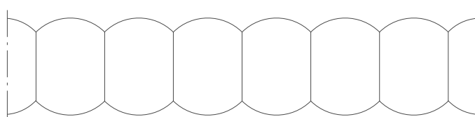
Gabions cloisonnés avec palplanches raccords à 120^\circ
