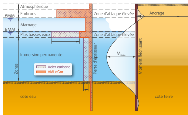
Perte d'épaisseur typique dans un milieu marin: acier carbone standard et AMLoCor®.
