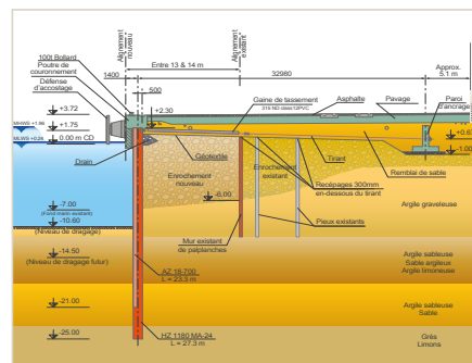
Coupe type d'un mur de quai
