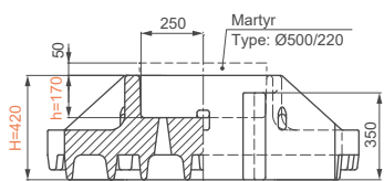
Coupe 1-1 (PUD 17-33) [mm]
