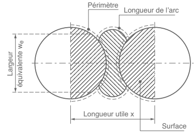
Gabions circulaires avec 1 arc
