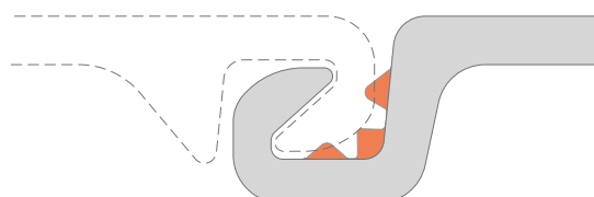
Joint MSP-1 extrudé dans une serrure libre.
