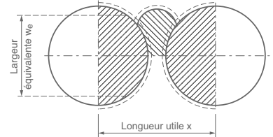
Gabions circulaires avec 1 arc
