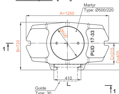
Vue en plan [mm]
