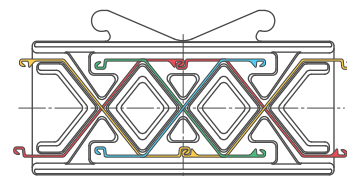
Vue de dessous
