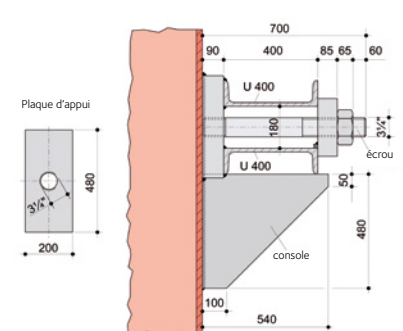
Détails d'exécution
