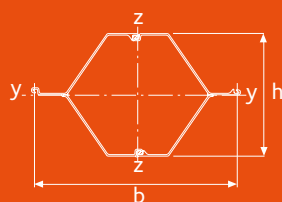
Caisson Z
