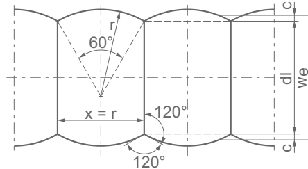
Gabions circulaires avec 1 arc
