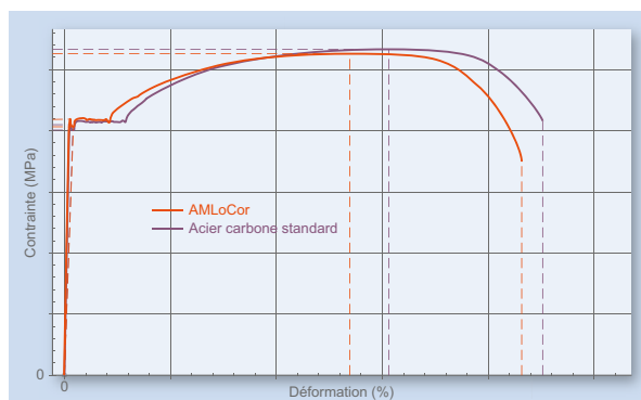
Diagramme contrainte / déformation d'une éprouvette d'acier carbone standard et AMLoCor®.
