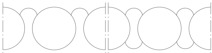
Gabions circulaires avec palplanches raccords à 35^\circ et un ou deux arcs de raccordement
